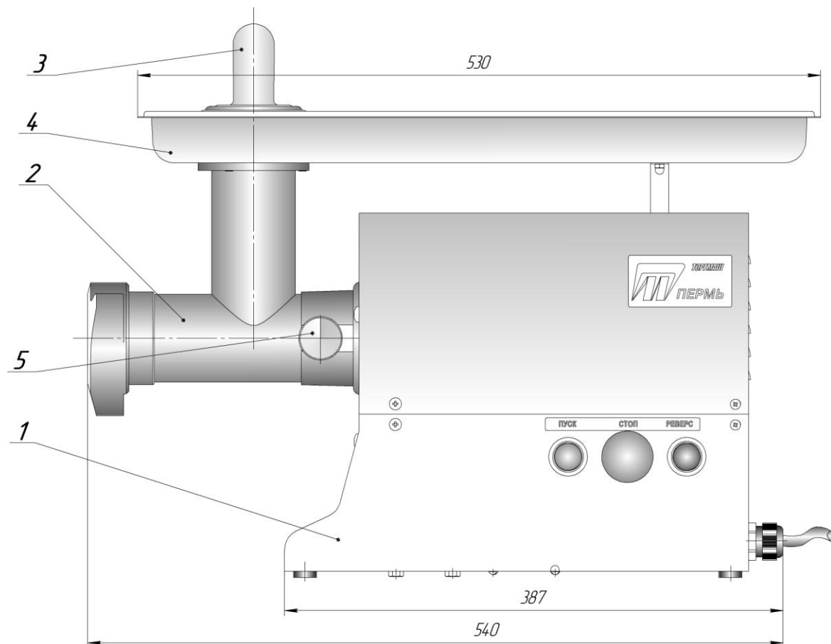
Рисунок 1 – Мясорубка М-150
