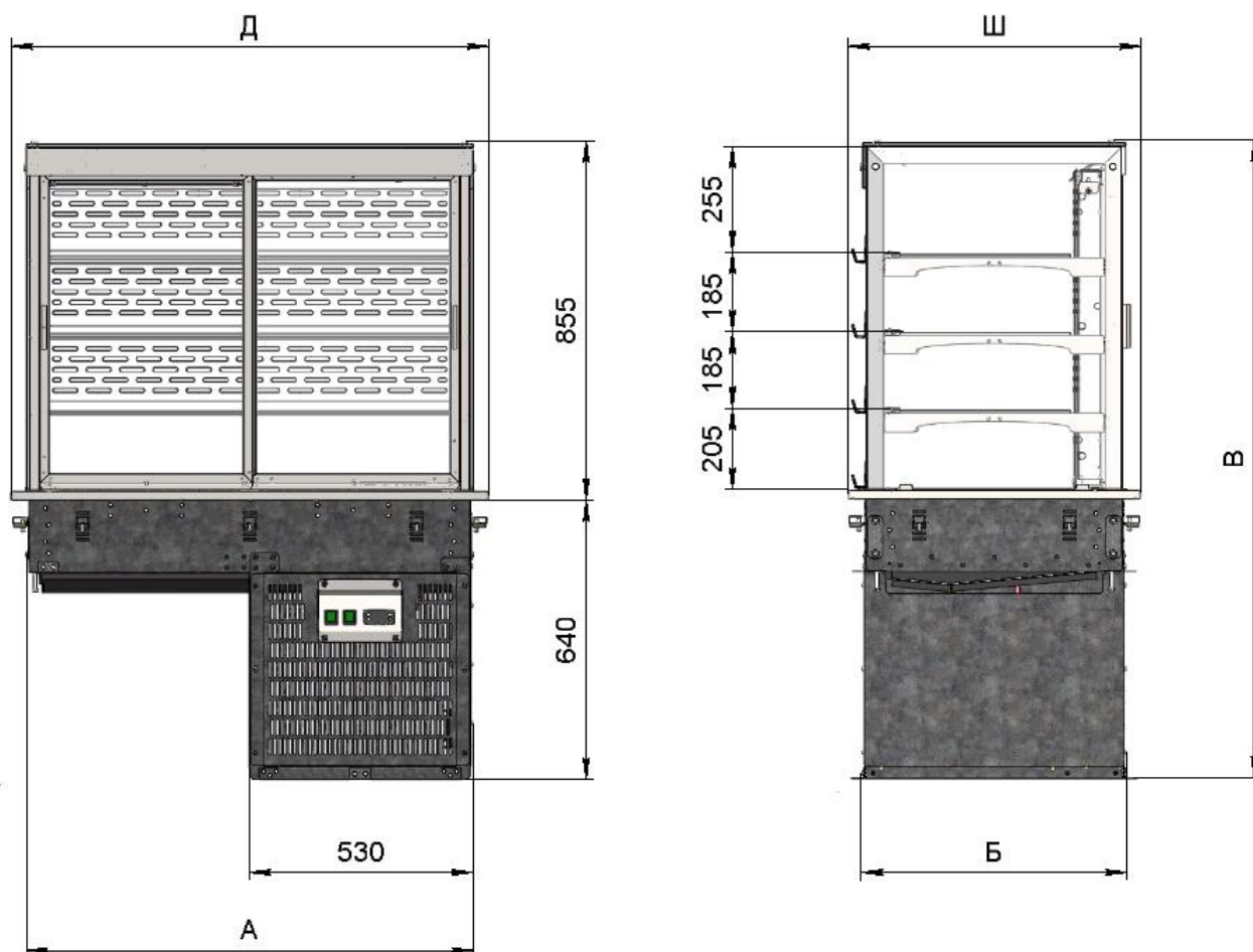
Рисунок 4. Основные габаритные размеры оборудования.
