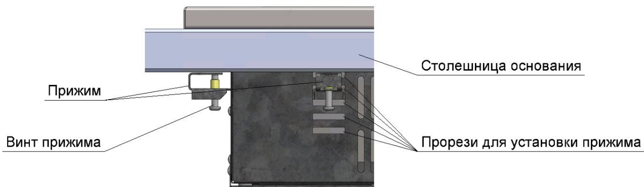
Рисунок 6. Установка прижимов.
