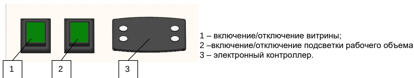
Рисунок 3. Внешний вид панели управления и назначение кнопок.
