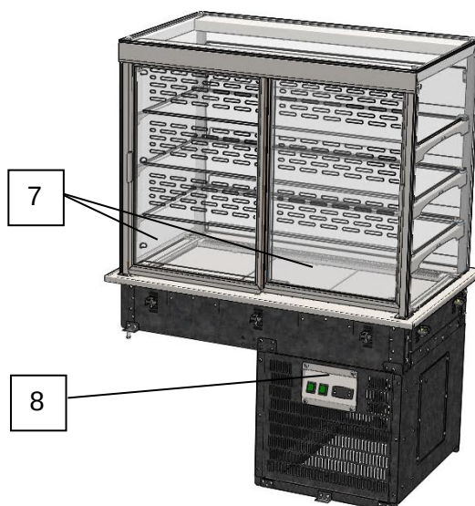
Рисунок 2. Вид витрины со стороны продавца.
