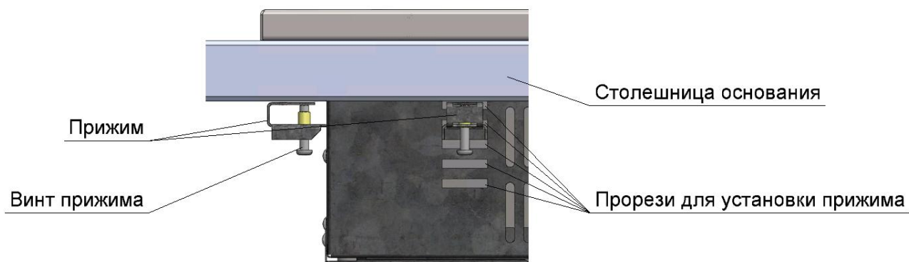
Рисунок 6. Установка прижимов.
