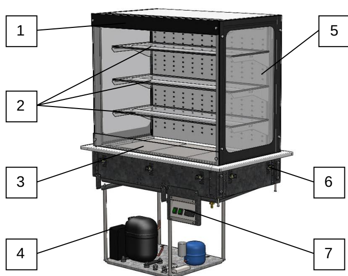
Рисунок 1. Вид витрины со стороны покупателя.
