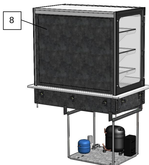
Рисунок 2. Вид витрины с обратной стороны.
