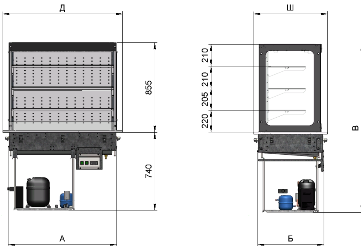
Рисунок 4. Основные габаритные размеры оборудования.
